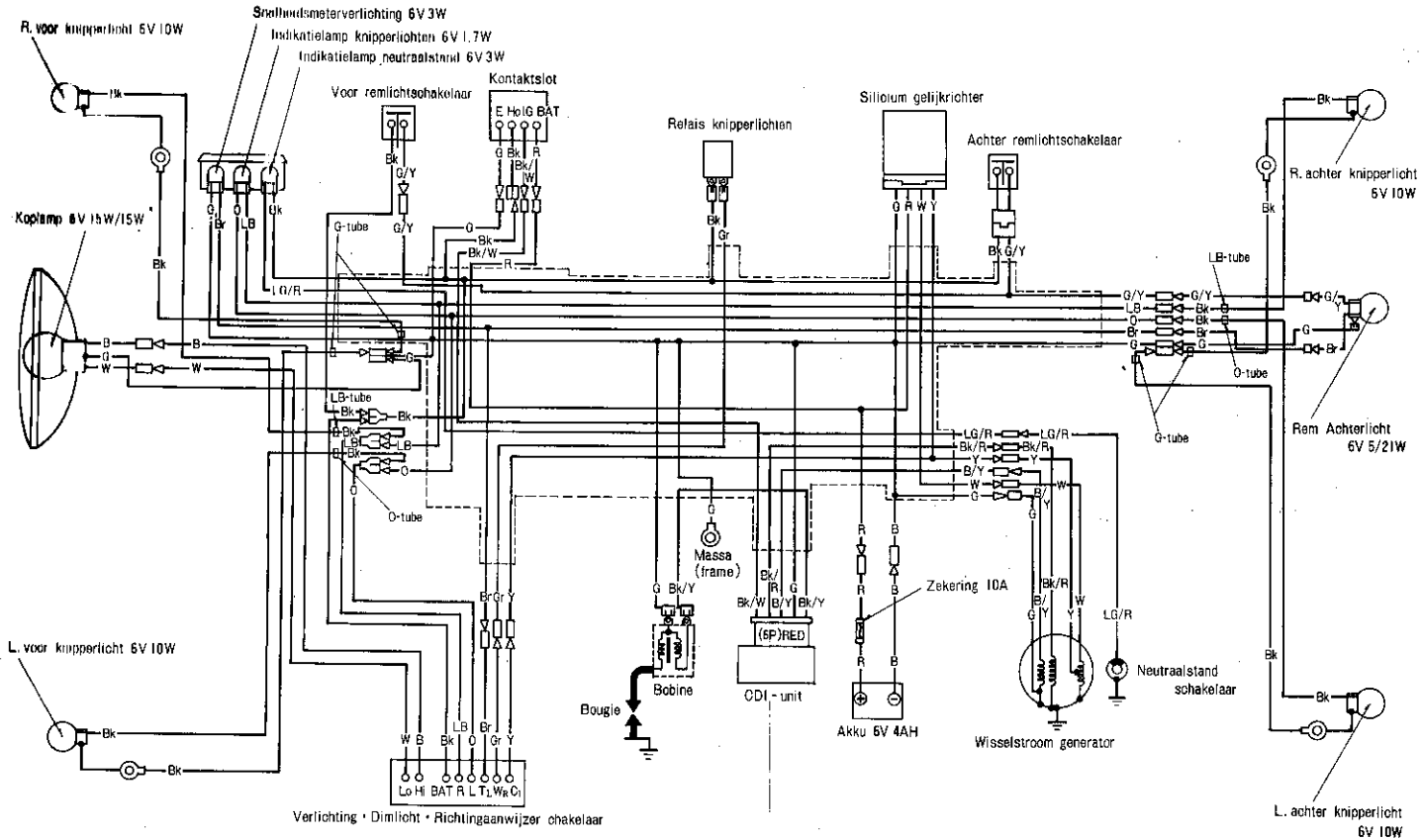
Schakelschema kontaktalot
